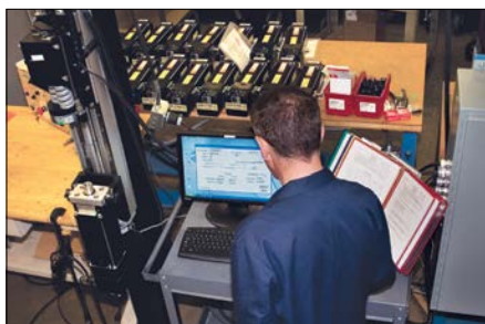
Prueba de funcionamiento de la unidad durante cientos de ciclos, cuantifica las carreras, la longitud, par bajo carga nula, entrada de corriente frente a la desviación de fuerza estándar.
